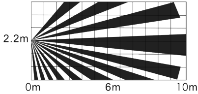
PIR DEDEKTÖR 15° 10m
